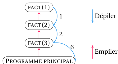
FIGURE 1 – Vision de la pile d'exécution de l'algorithme factoriel récursif ?? pour le calcul de 3!
